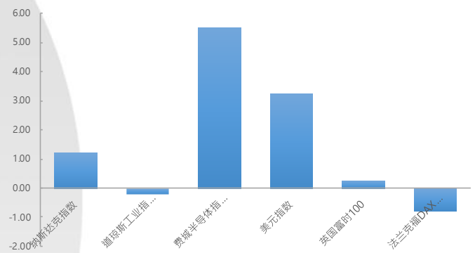
全球主要金融市场指数日涨跌幅%
