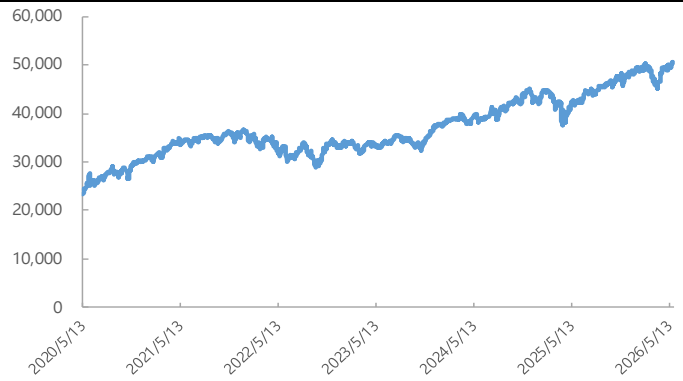
道琼斯工业平均指数（日）
